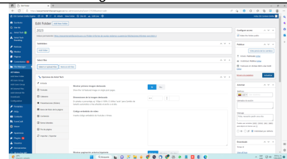
Imagen 43 Actualizar
