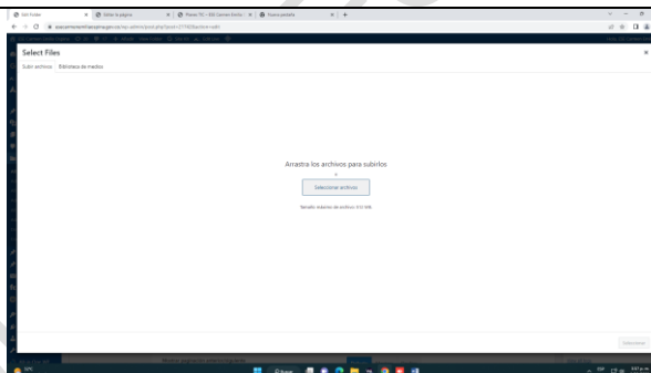
Imagen 32 Seleccionar archivo
