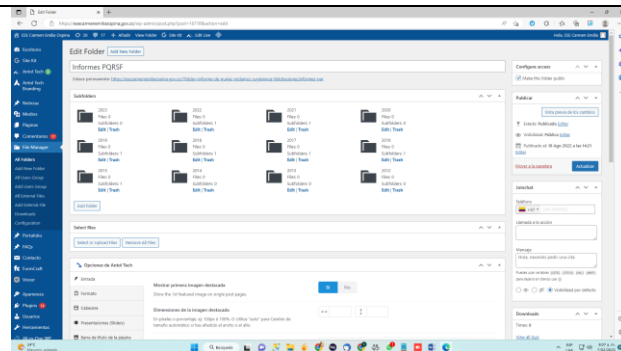
Imagen 22 Año respectivo
