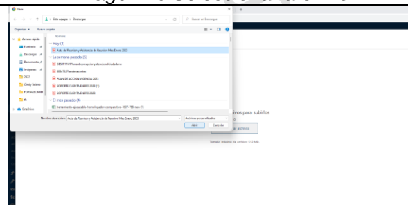
Imagen 17 Abrir
