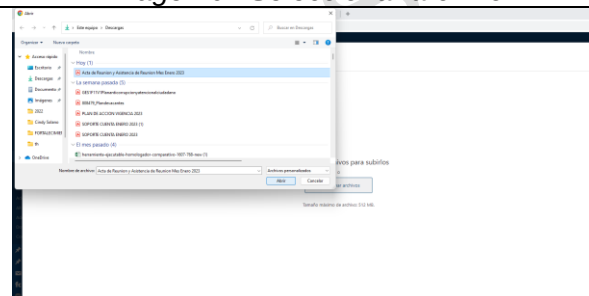
Imagen 65 Abrir
