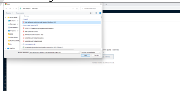
Imagen 9 Abrir
