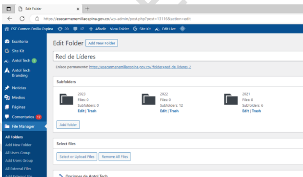
Imagen 62 Año respectivo
