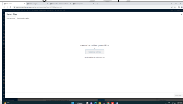
Imagen 56 Seleccionar archivo
