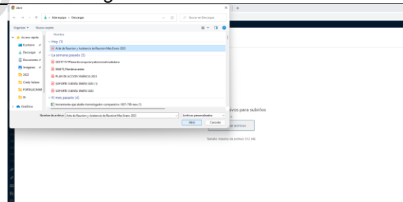
Imagen 33 Abrir
