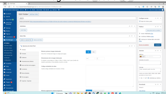
Imagen 51 Actualizar
