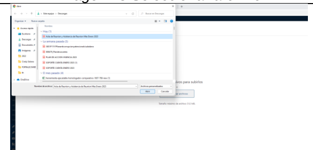
Imagen 49 Abrir
