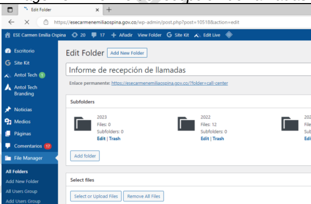
Imagen 38 Año respectivo
