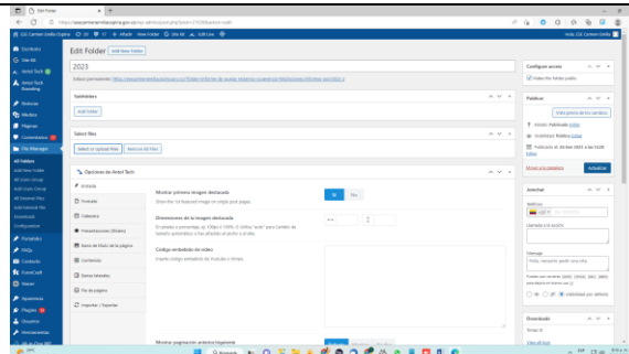
Imagen 35 Actualizar
