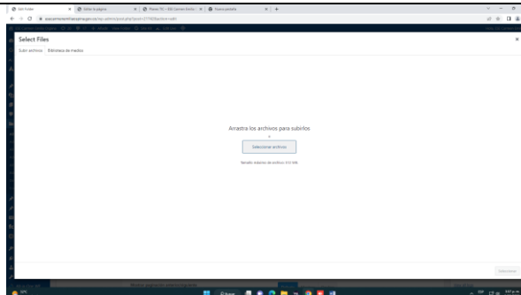
Imagen 40 Seleccionar archivo
