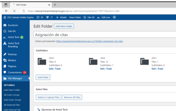
Imagen 46 Año respectivo
