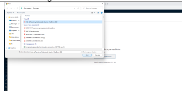
Imagen 25 Abrir
