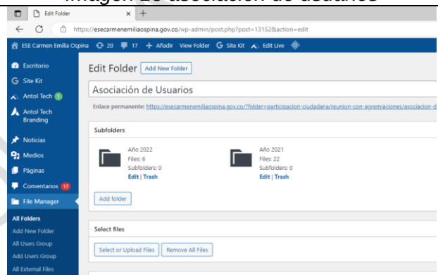
Imagen 14 Año Respectivo
