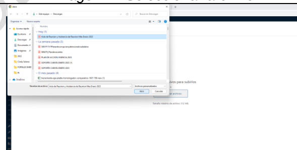
Imagen 73 Abrir
