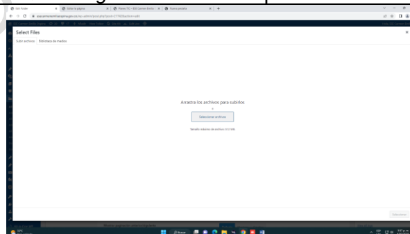
Imagen 24 Seleccionar archivo
