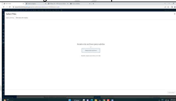
Imagen 8 Seleccionar archivo
