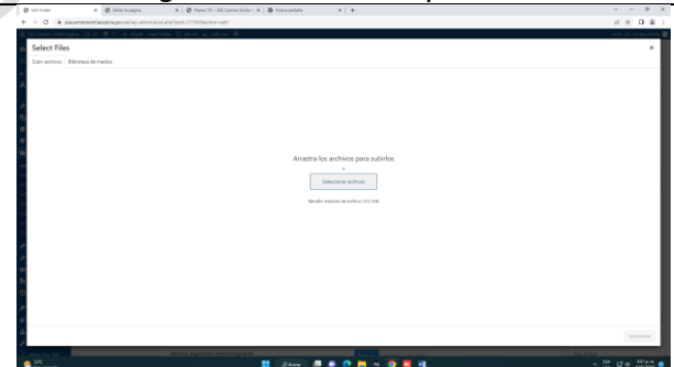
Imagen 48 Seleccionar archivo
