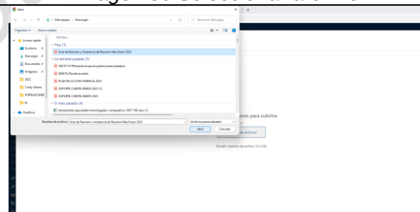
Imagen 57 Abrir
