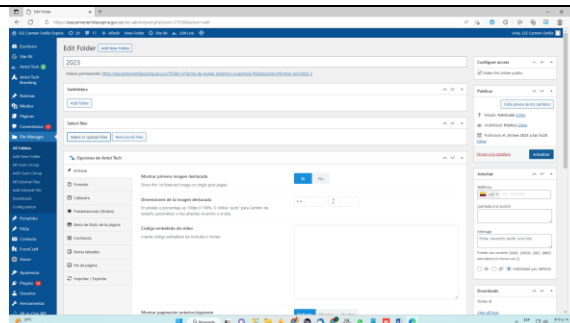
Imagen 59 Actualizar
