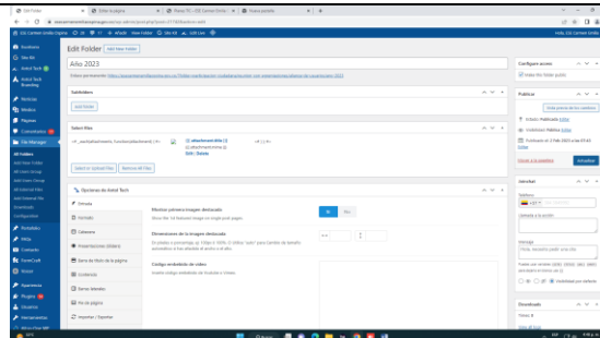
Imagen 11 Actualizar
