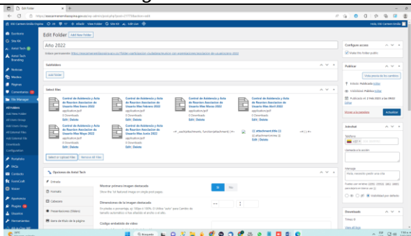
Imagen 19 Actualizar
