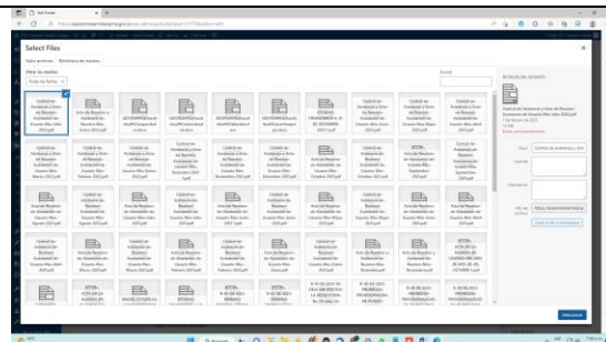
Imagen 50 Seleccionar
