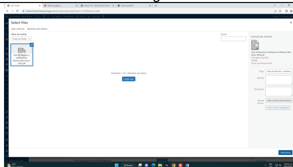
Imagen 10 Seleccionar
