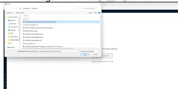
Imagen 41 Abrir
